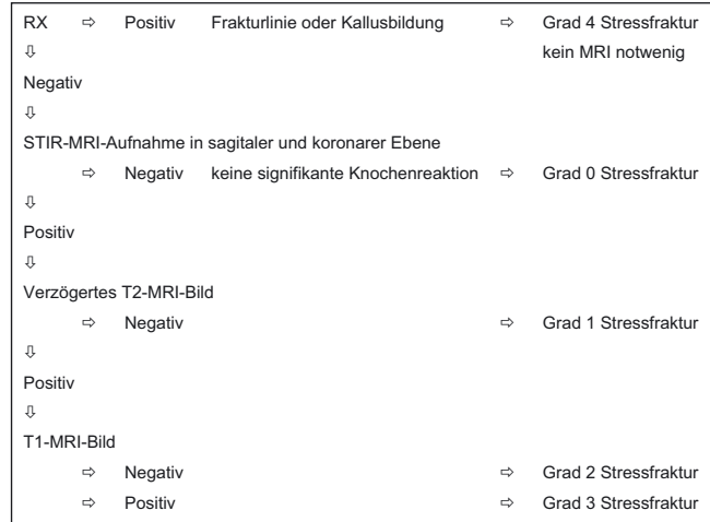
Abbildung 3: Diagnostik Algorithmus.
